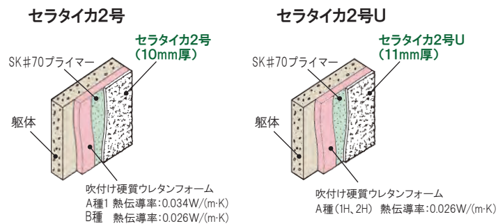
セラタイカ2号/2号U
